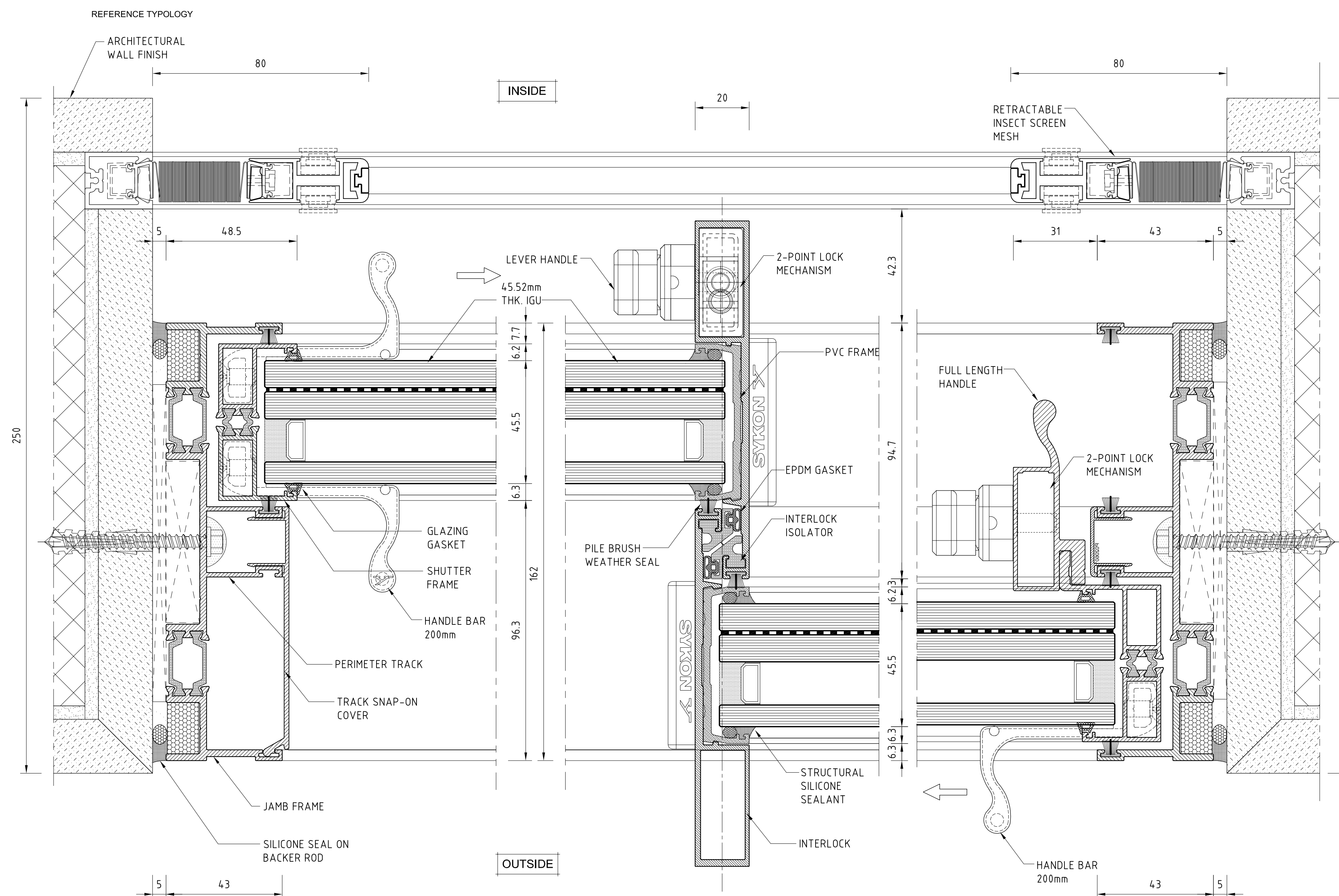
JAMB DETAIL
